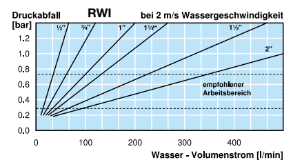
RWI-02...-10B/C/E/F/G
